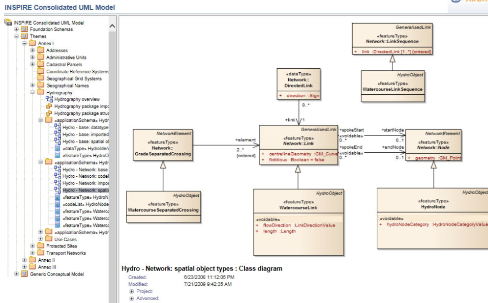
Abbildung 21 - UML-Diagramm
